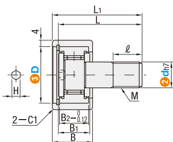
■ (d8 · 10) 头部内六角孔
