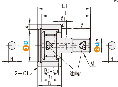
■ (d12 · 16) 头部螺纹部内六角孔
