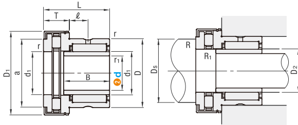
BAKXRZ (带止推滚针滚针轴承)
