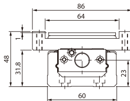
剖面:A-A
