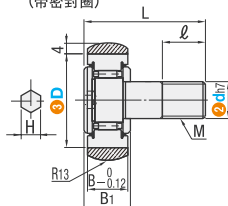
■ 头部内六角孔(d5~10) (带密封圈)
