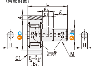
■ 头部螺纹部内六角孔(d12~16) (带密封圈)
