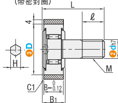
■ 头部内六角孔(d5~10) (带密封圈)
