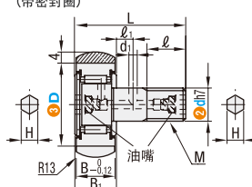
■ 头部螺纹部内六角孔(d12~16) (带密封圈)
