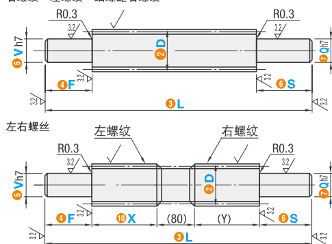
右螺纹·左螺纹·细螺距右螺纹
