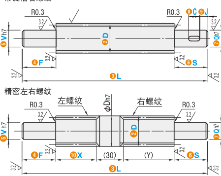
带键槽右螺纹
