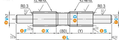
左右螺纹
