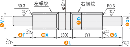
精密左右螺纹
