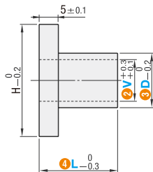
肩型轴环
