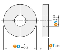
垫圈
