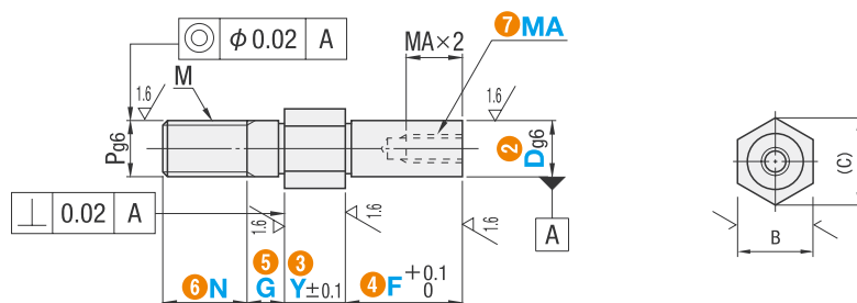
螺纹长度 指定型
