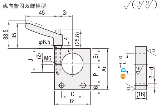
纵向紧固双螺栓型
